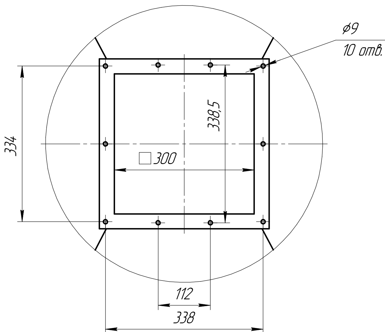
Б(1:5)
