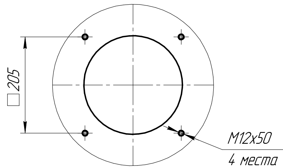
B(1:5)
